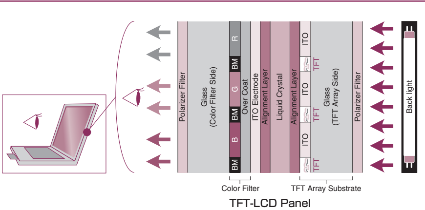
Cross section 断面図
