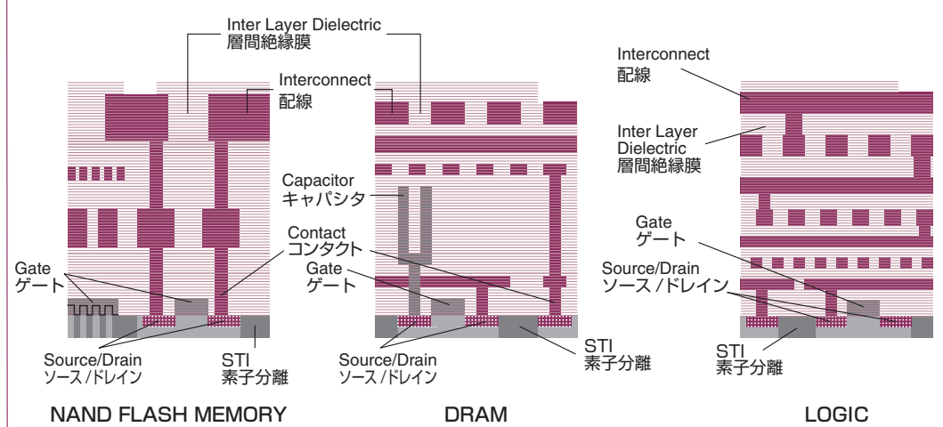
Cross section 断面図
