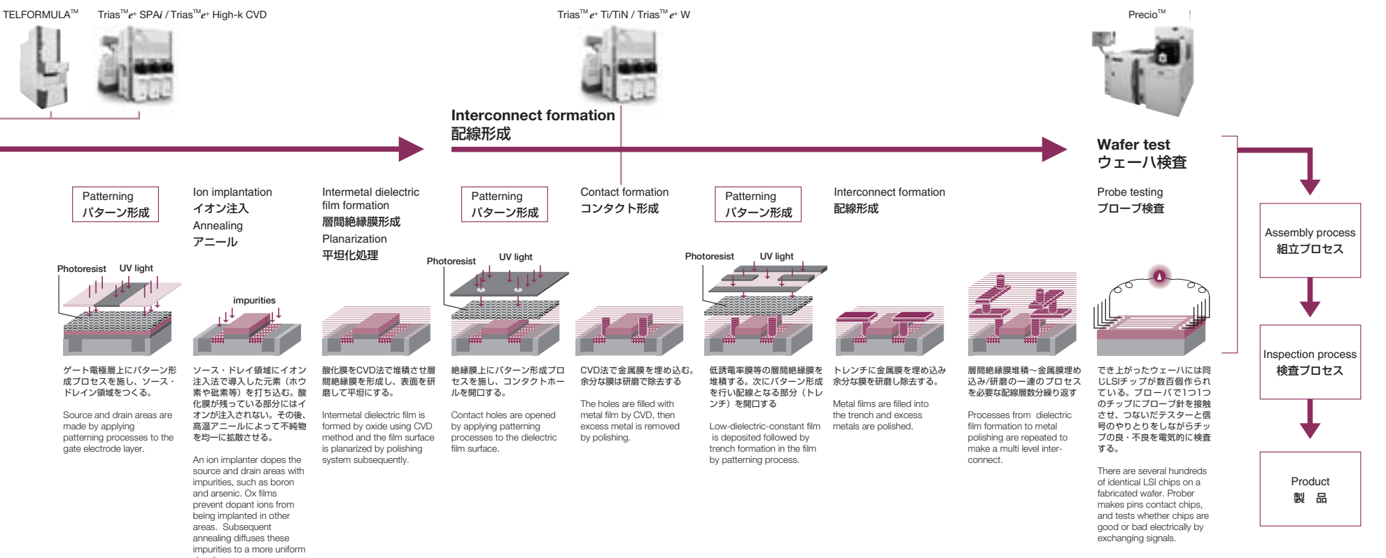
Cross section 断面図
