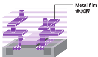
Plasma Etch System プラズマエッチング装置 Tactras™ Plasma Etch System プラズマエッチング装置 Episode™ UL
